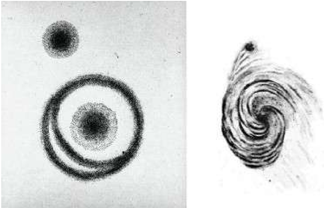
Rys. 1. Po lewej: Szkic M51 (znanej również jako Galaktyka Wir) narysowany przez Johna Herschela w 1833 roku. Po prawej: Ta sama galaktyka naszkicowana przez Williama Parsona w 1845 roku. Kolory są tu odwrócone. Teleskop Parsona pozwolił mu zobaczyć więcej szczegółów tej galaktyki, niż dostrzegał Herschel. Źródło: 'A newly-discovered accurate early drawing of M51, the whirlpool nebula'. Journal of Astronomical History and Heritage, William Tobin.
